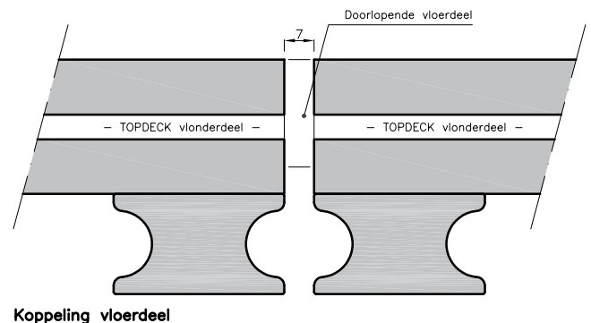
Koppeling vloerdeel
