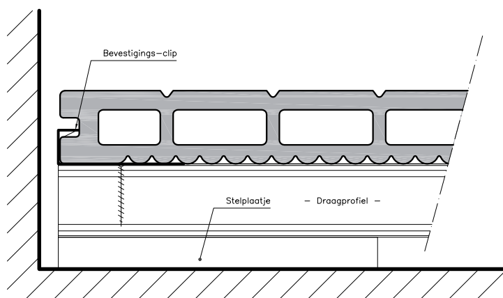
Bevestiging eerste deel
