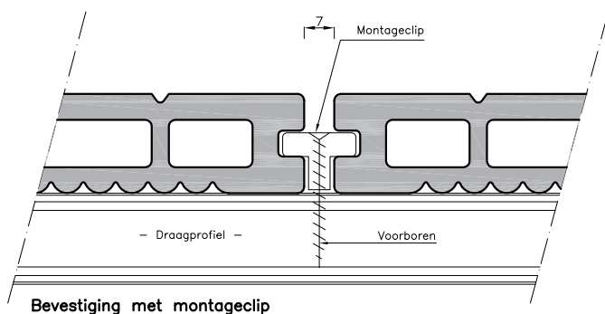
Bevestiging met montageclip
