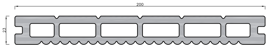
Topdeck XL vlonderdeel
